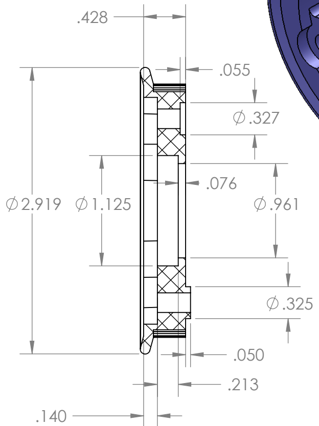
SECTION A-A
