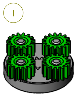
4:1 PLANET, 5:1 SUN
