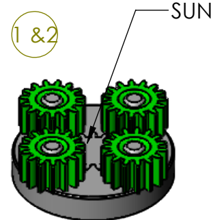
4:1 PLANET, 4:1 SUN
