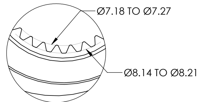
DIN 5481-7x8(z=28) DETAIL A SCALE 7 : 1
