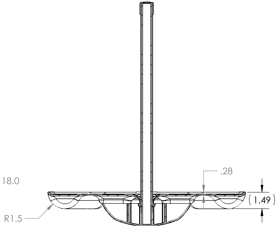
SECTION A-A
