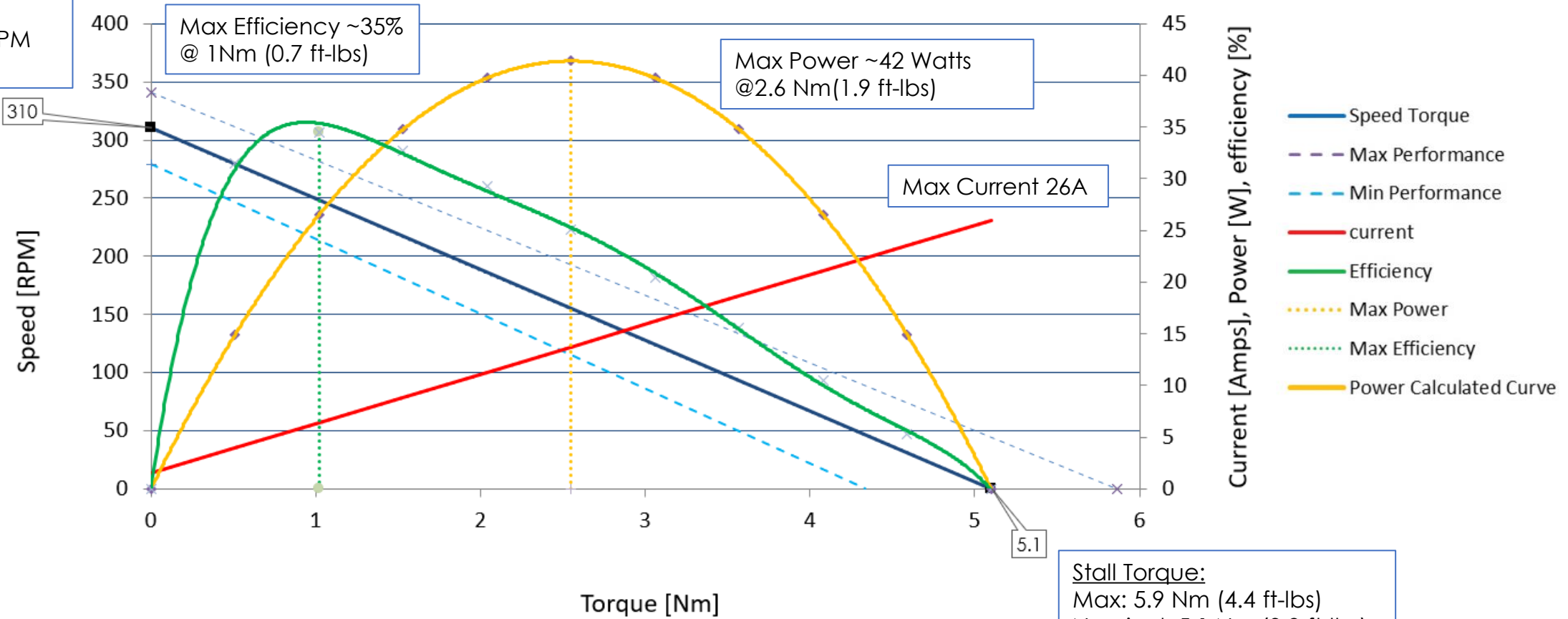
JE PLG motor for FRC JE-PLG-410 @12 V , 0 ohms
