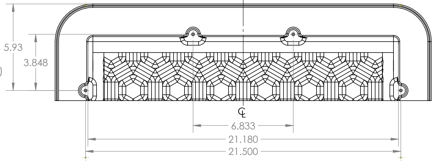
SECTION B-B SCALE 1 : 4
