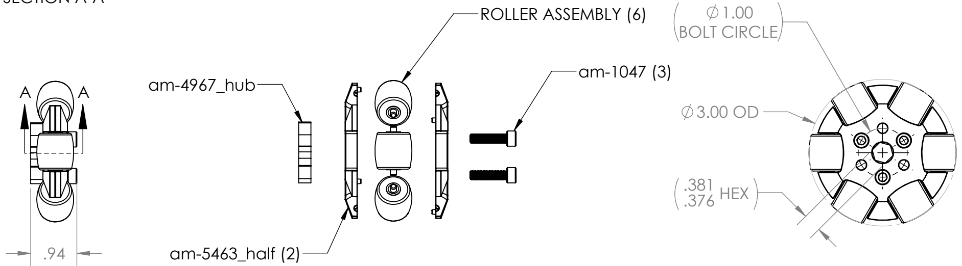
SECTION A-A
