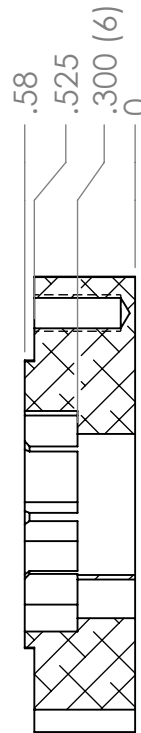
SECTION A-A
